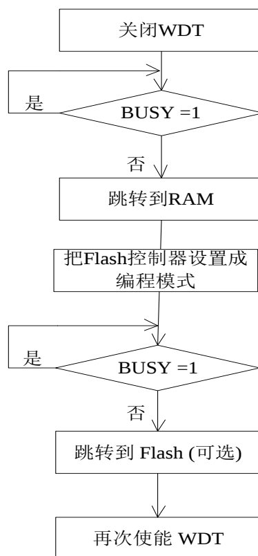
Figure 10-7 RAM 中运行程序进行 Flash 编程
