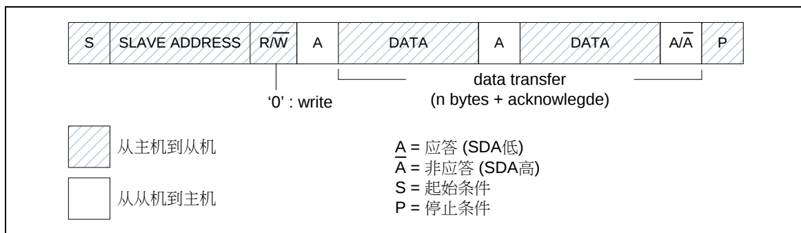
Figure 26-3 主机向从机传输数据
