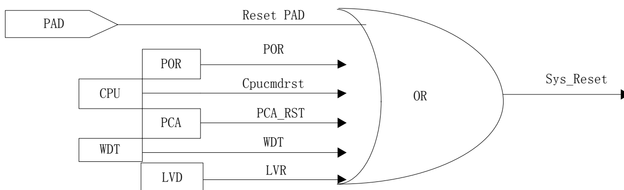
ure 14-1 复位源构成
