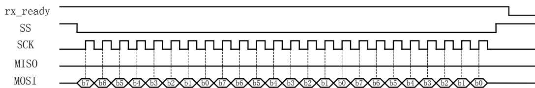
Figure 25-6 SPI 从模式时数据接收状态时序图
