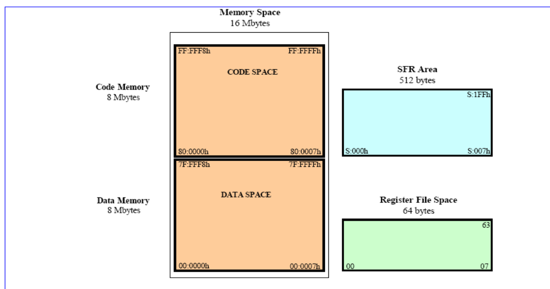
Figure 7-2 80251 内存空间分布图
