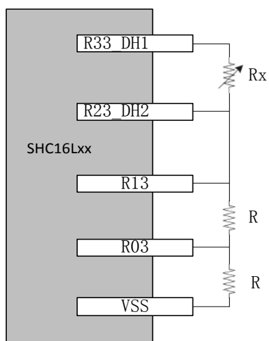
1/2 电阻分压型
