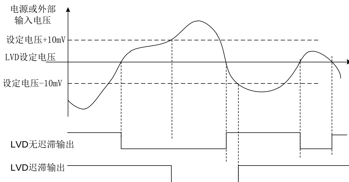
Figure 30-3 LVD 迟滞响应
