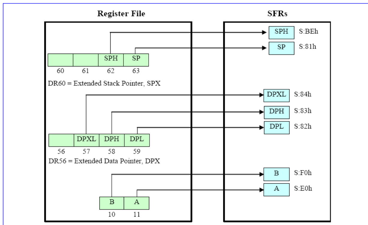
Figure 7-11 专用寄存器在寄存器文件组位置以及相对应的SFR地址
