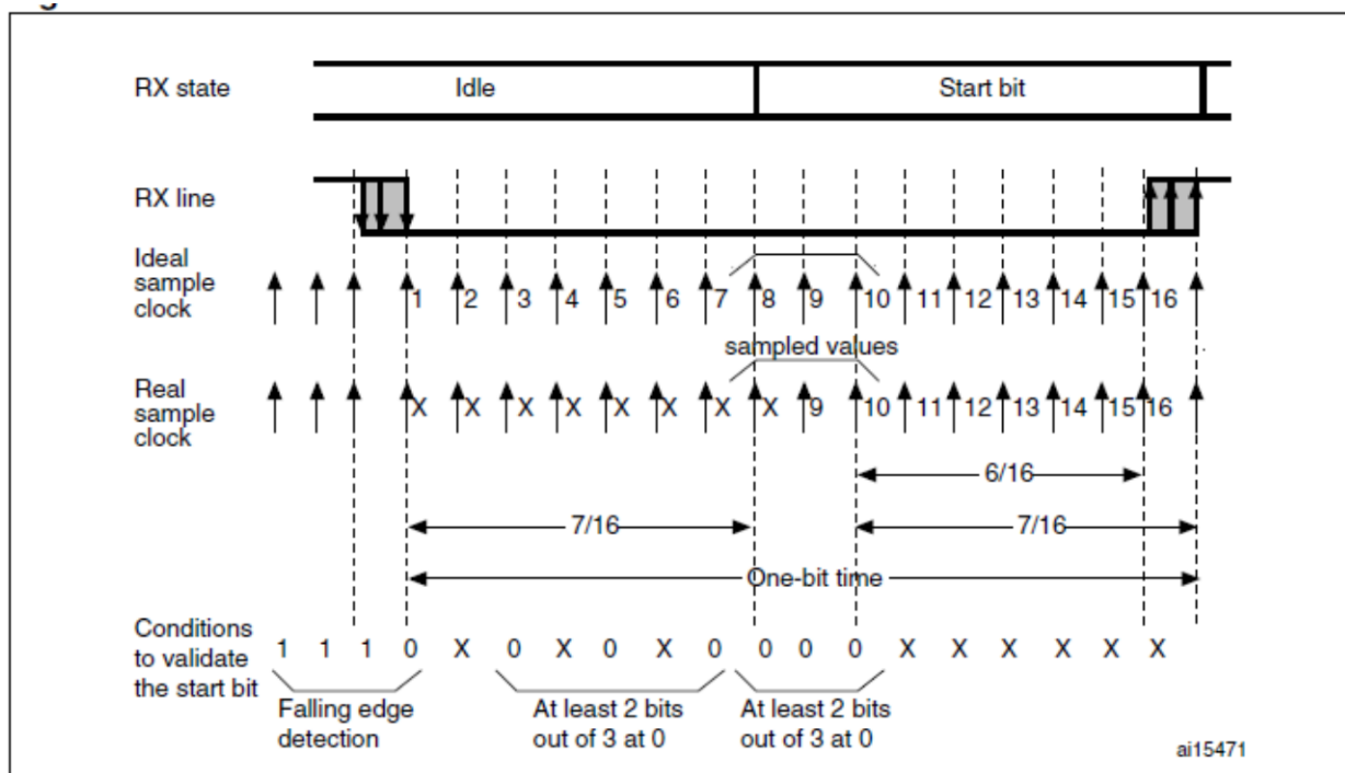
Figure 27-4 采样判决方式
