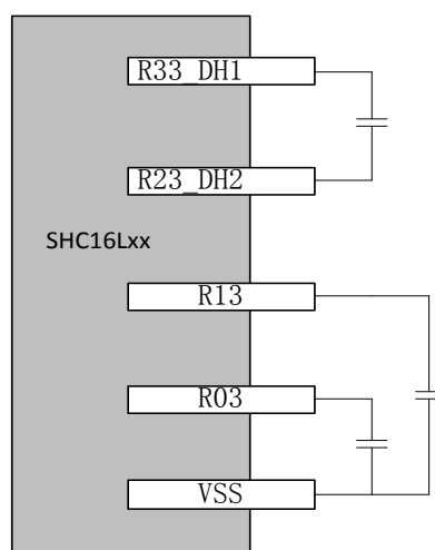
1/3 电荷泵型
