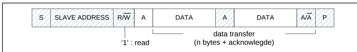
Figure 26-4 主机由从机读取地址
