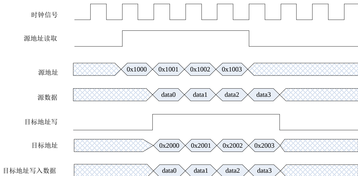
Figure 11-1 DMA 并行操作时序图
