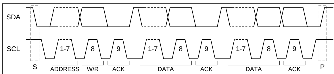
Figure 26-2 I 2 C 传输协议
