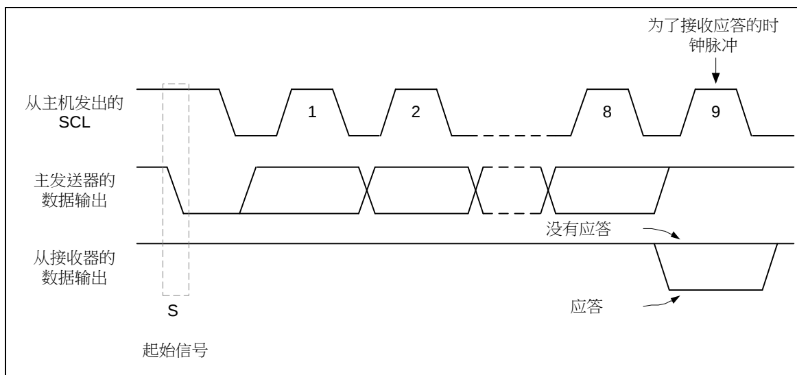
Figure 26-7 I²C 总线上应答信号
