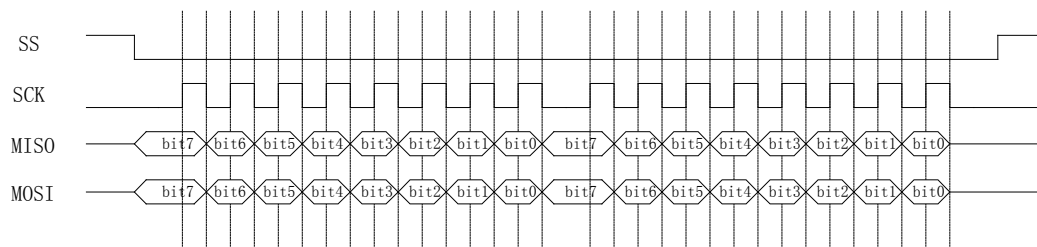
Figure 25-4 SPI 主模式时全双工方式时序图
