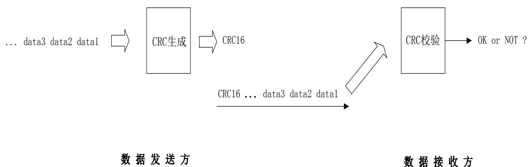
Figure 23-1 CRC 数据传输模型
