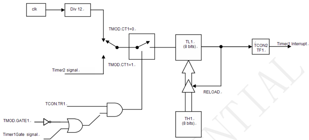
Figure 17-5 溢出自动加载 定时/计数器 工作模式
