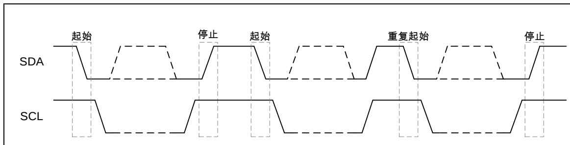
Figure 26-5 START 和 STOP 条件
