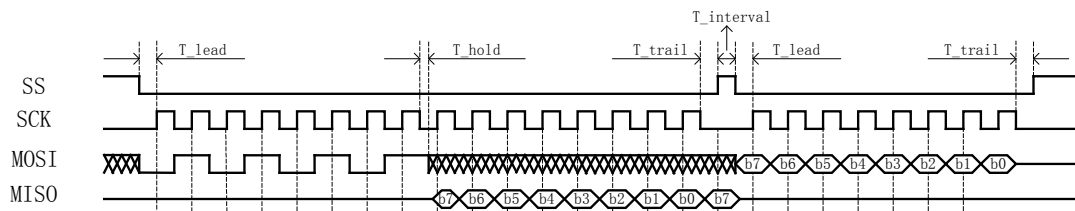
Figure 25-11 对主设备 SPI 的时序要求
