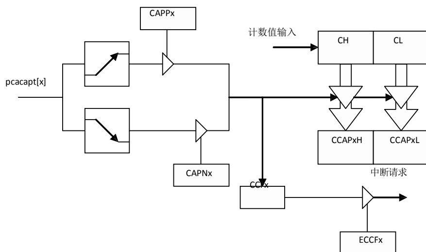
Figure 18-3 PCA 16位捕获模式
