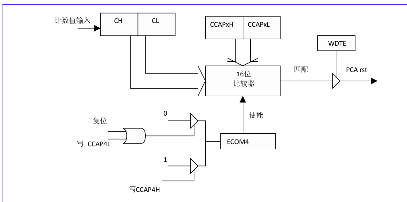
Figure 18-5 PCA WDT功能
