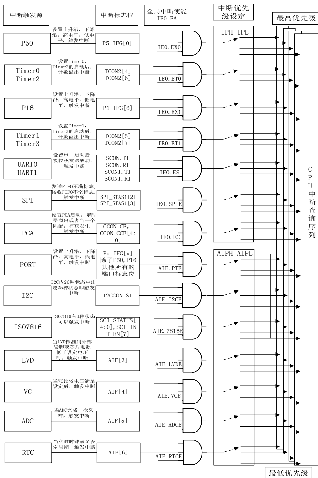
Figure 15-1 中断框图
