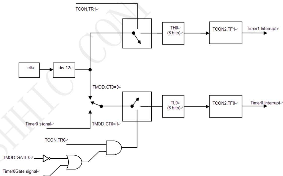
Figure 17-6 2个8位定时/计数器工作模式
