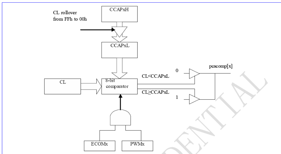
Figure 18-7 PCA 8位 PWM 功能模块
