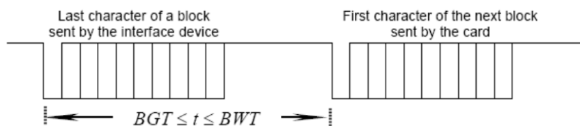
Figure 27-3 ISO7816 块保护时间
