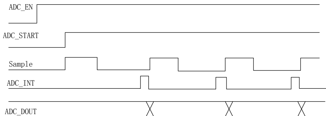
Figure 28-3 ADC 连续采样过程
