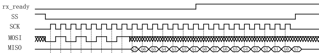
Figure 25-5 SPI 从模式时报告状态时序图
