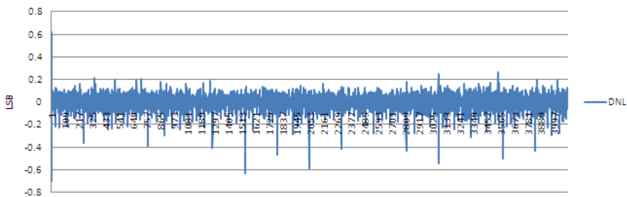
DNL
