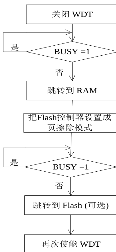
Figure 10-5 RAM 中运行程序进行 Flash 页擦除
