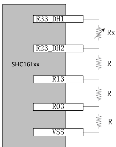
1/3 电阻分压型
