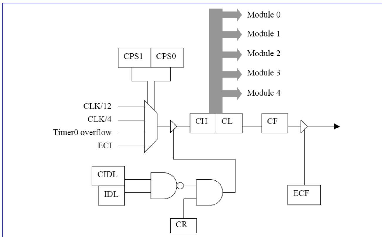
Figure 18-2 PCA定时/计数模式
