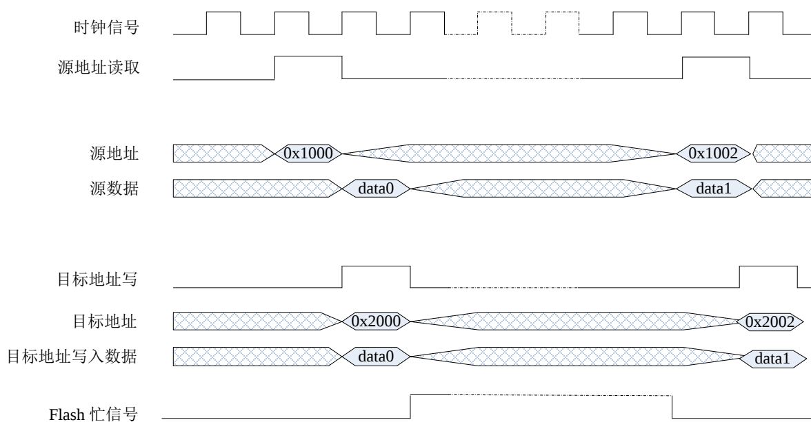
11-3 DMA 串行等待Flash时序模式图
