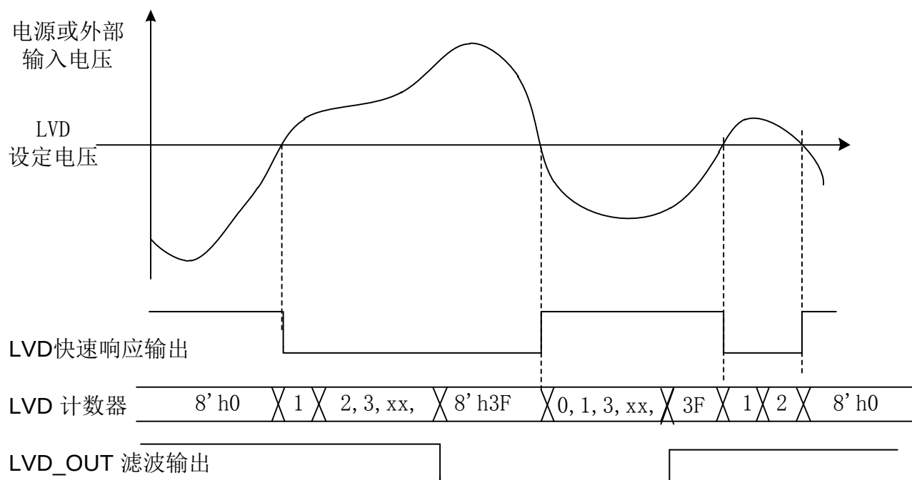
Figure 30-2 LVD 滤波响应时间
