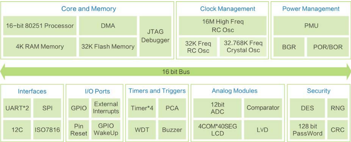
Figure 2-1 HC16Lxx 功能模块简介图
