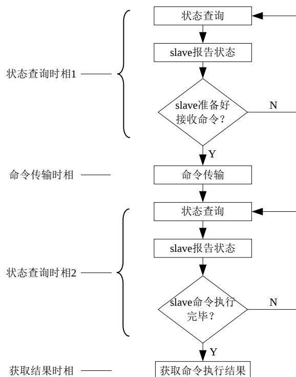
Figure 25-10 SPI 主从 SPI 通讯流程
