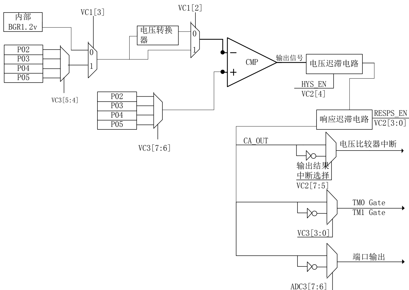
Figure 29-1 模拟电压比较器框图
