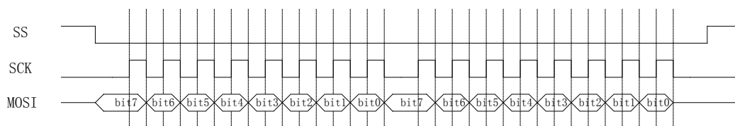
Figure 25-2 SPI 主模式时发送方式时序图
