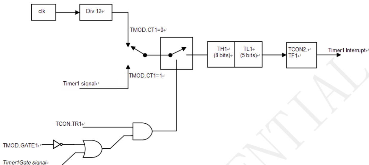
Figure 17-3 13位计数器/定时器工作模式
