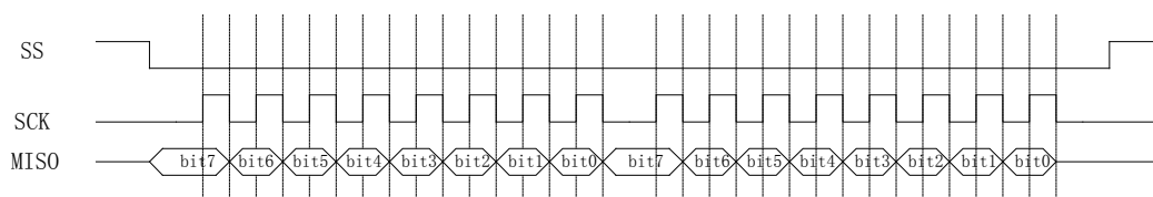
Figure 25-3 SPI 主模式时接收方式时序图
