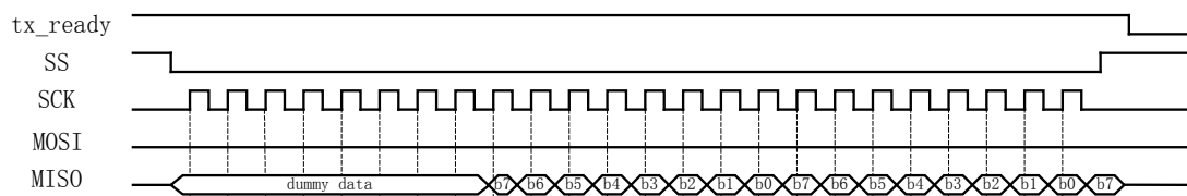
Figure 25-7 SPI 从模式时数据发送状态时序图
