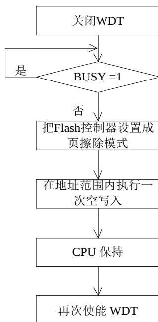
Figure 10-4 Flash 中运行程序进行 Flash 页擦除
