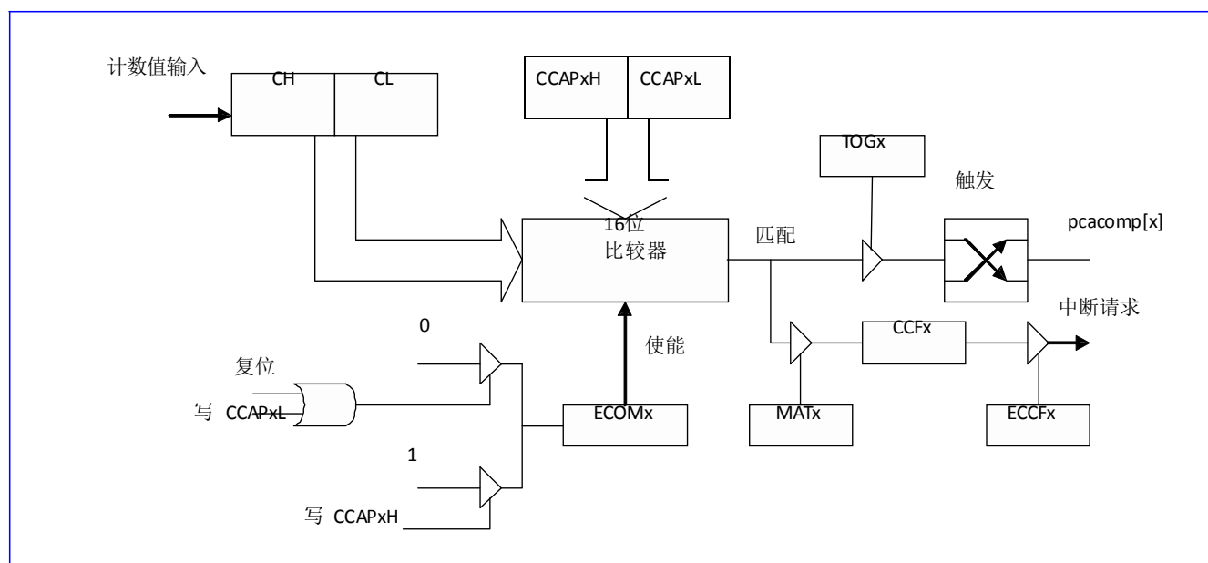
Figure 18-4 PCA 软件计数器以及高速输出模式
