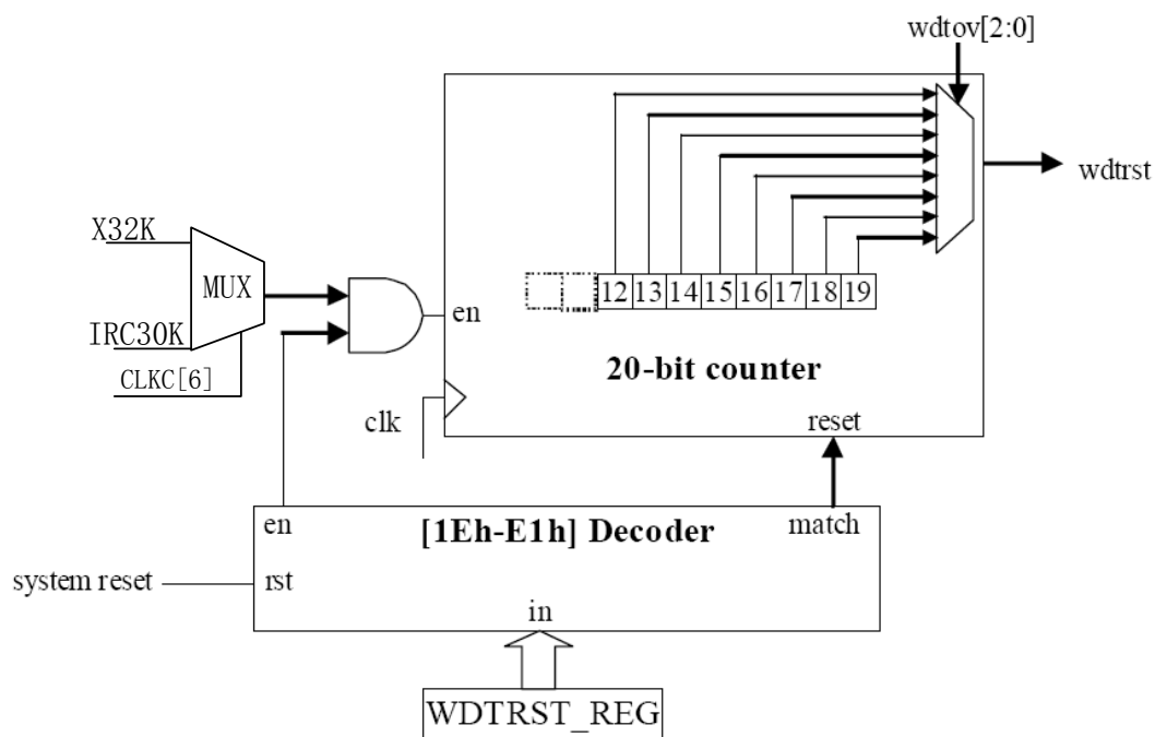
Figure 19-1 看门狗功能模块
