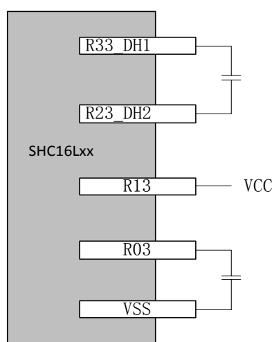
1/2 电荷泵型
