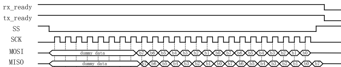
Figure 25-8 SPI 从模式时全双工状态时序图
