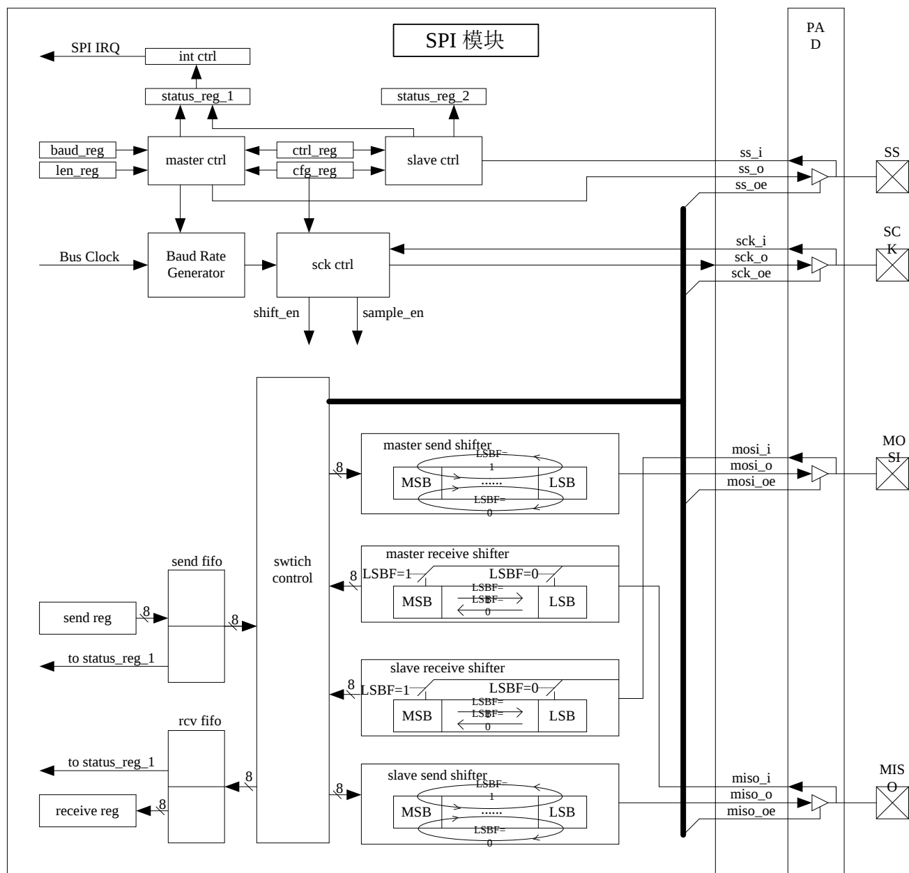
Figure 25-1 SPI 架构框图
