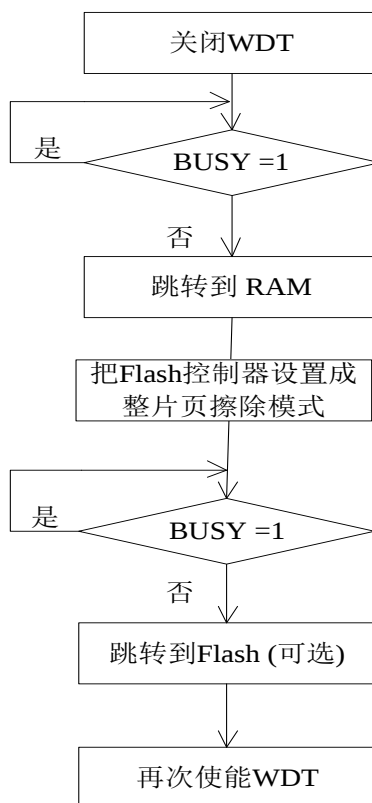
Figure 10-3 RAM 中运行程序进行 Flash 整片页擦除
