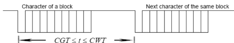
Figure 27-2 7816 字符等待时间
