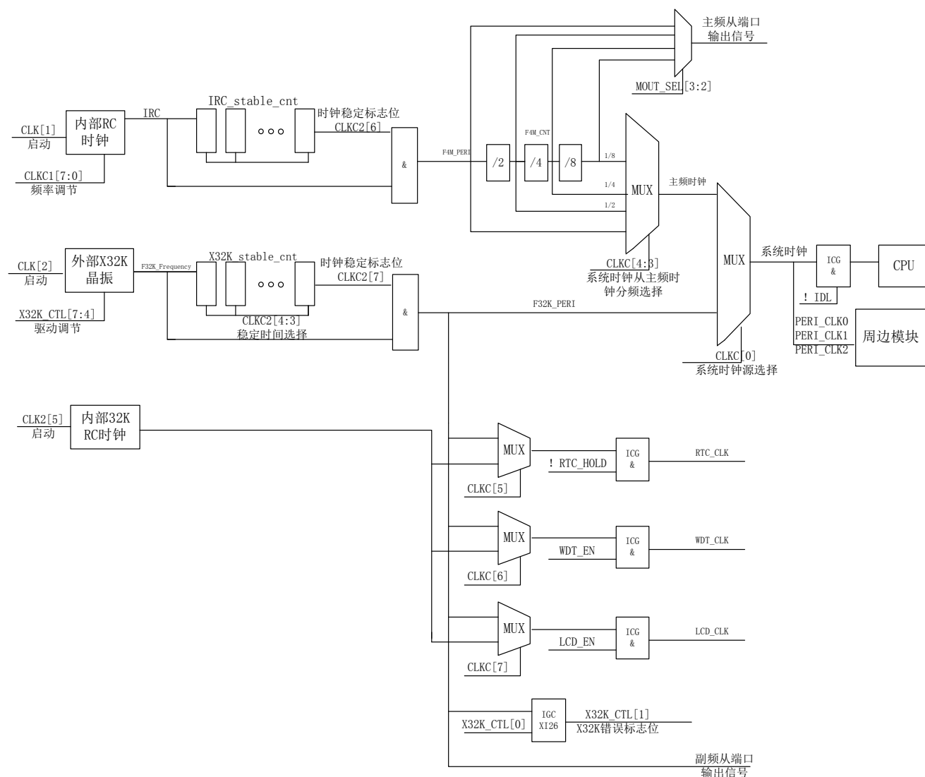
Figure 13-1 HC16Lxx 时钟分配图
